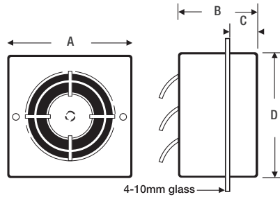
Dimensions - WF
